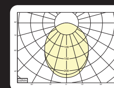
61220BL.16.30 16w 3000k 2280lm ηLB 100%
