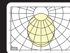
61197WM.1430D 14w 3000k 1610lm ηLB 100%
