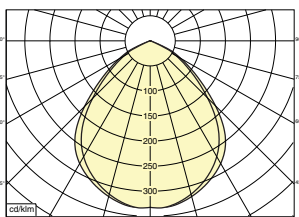
23008W.31D.RGB 31w 2280lm ηLB 76%
