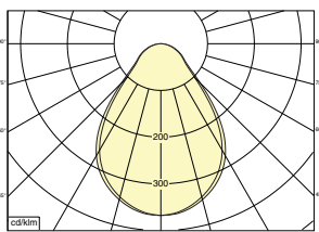
62006W.00-W 12w 3000k 1610lm ηLB 74%
